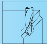
Umfangsfräsen und Fasen
